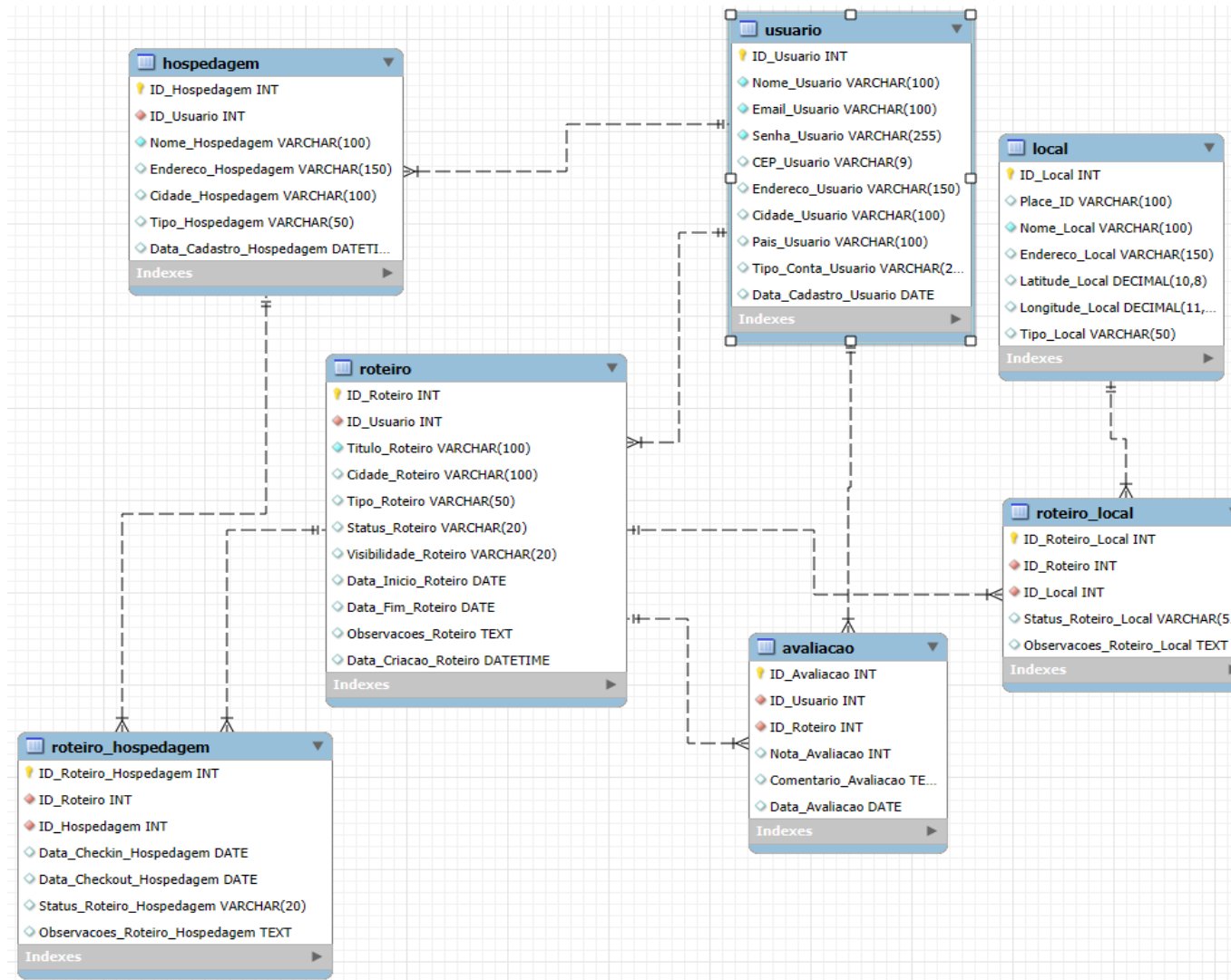
Figura 34 - Modelo físico DER
