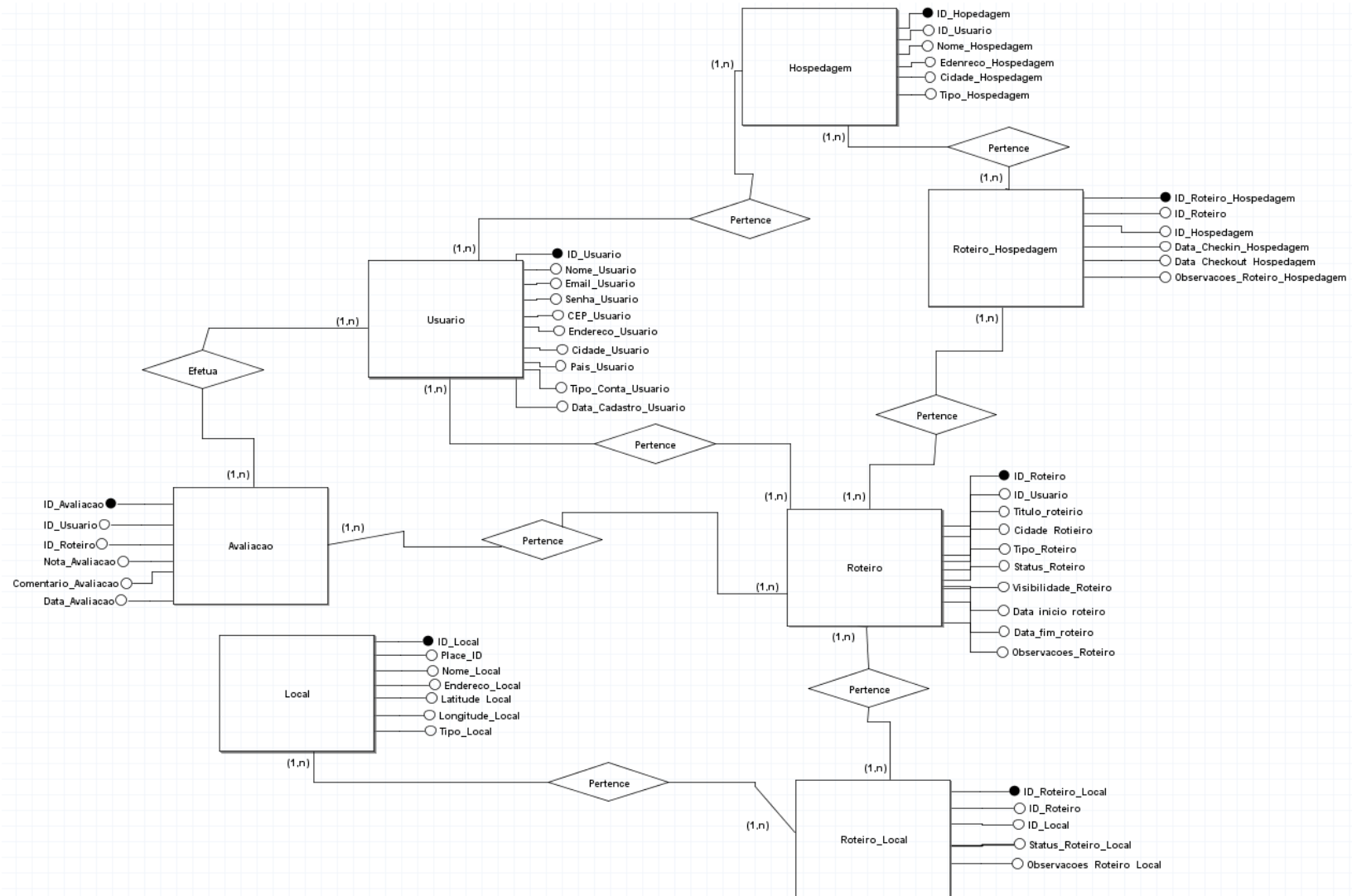
Figura 33 - Diagrama de entidade e relacionamento
