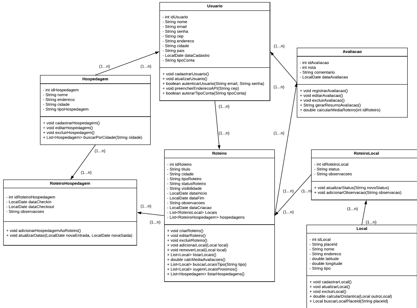
Figura 15 - Diagrama de Classes
